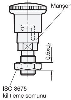
Tip AK / ARK Geri çekilmiş ve kilitli piston
