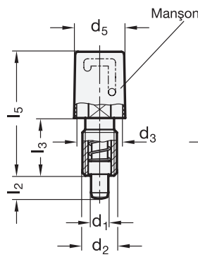
Tip B Dışarı çıkmış piston
