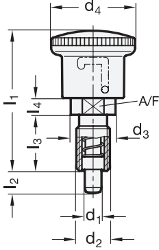
Tip A / AR Dışarı çıkmış piston
